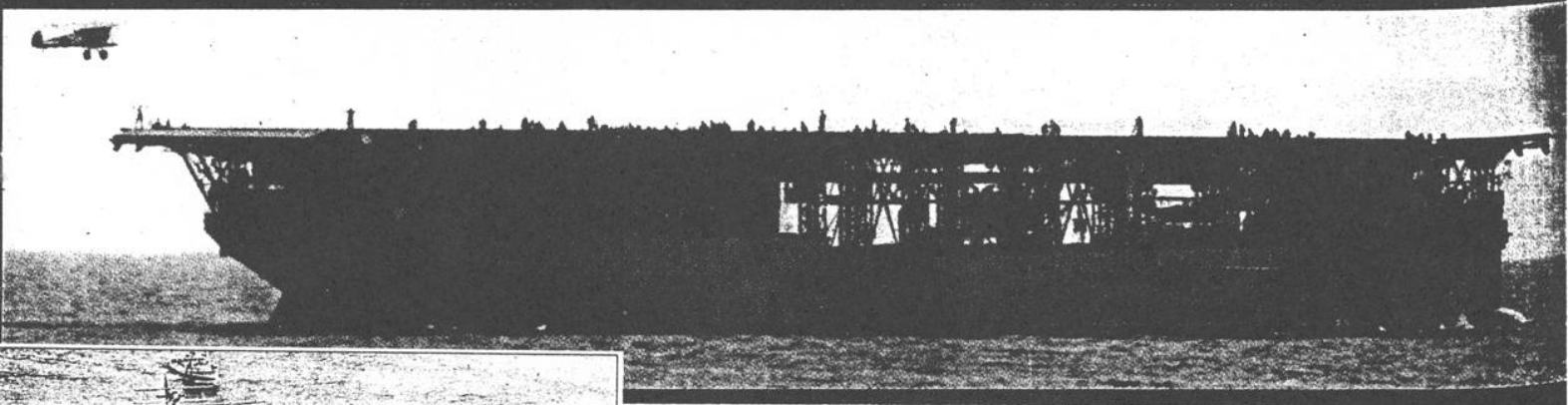
着艦機が進入中のラングレー。基準排水量11,950トン、全長165.3メートル、速力15ノットの小型低速空母だったが搭載機は33機と多かった。
